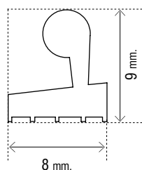
Art. OMTACC5
