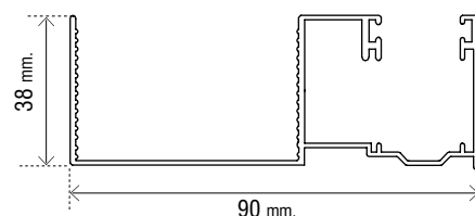
Art. OMTGU9038
