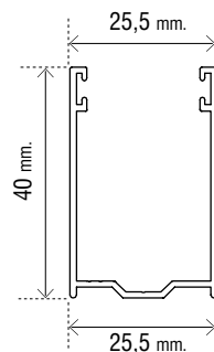
OMTGU2540
