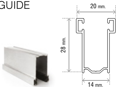
Guida in alluminio estruso 14 x 28 mm
