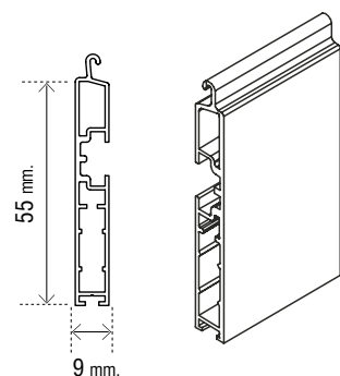
Terminali in alluminio estruso 9 x 55 mm
