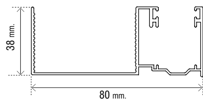
Art. OMTGU8038 Guide con predisposizione zanzariere 80 x 38 mm.
