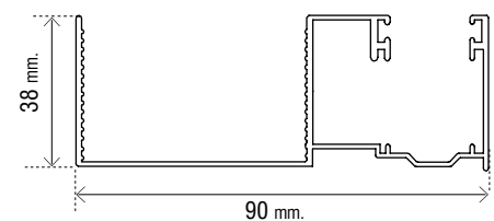
Guide con predisposizione zanzariere 90 x 38 mm.
