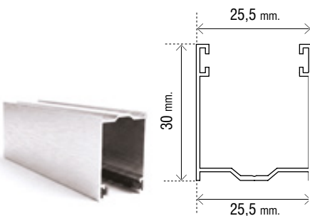
Guida in alluminio estruso 25 x 30 mm
