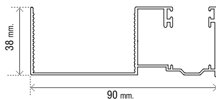
Art. OMTGU9038 Guide con predisposizione zanzariere 90 x 38 mm.
