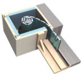
cod. A03 Cassonetto in multistrato di pioppo da 18mm., verniciato con cementite, guarnizione sul perimetro dello sportello, coibentato internamente, sportello avvitato con tappi bianchi sulle viti, completo di predisposizione per cappotto esterno. Cassonetto certificato ISTEDIL
