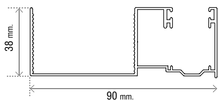
Art. OMTGU9038 Guide con predisposizione zanzariere 90 x 38 mm.
