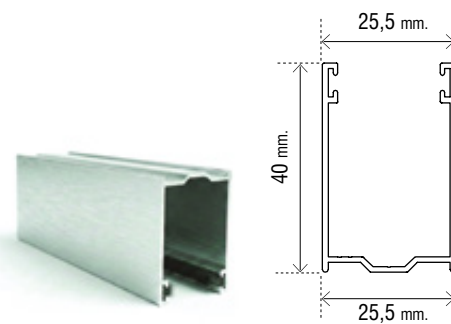
Guida in alluminio estruso 25 x 40 mm
