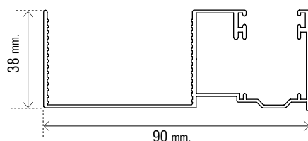
Art. OMTGU9038
