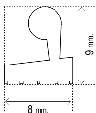
Art. OMTACC5 Terminale in Pvc rigido 8 x 9 mm.
