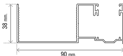
Art. OMTGU9038
