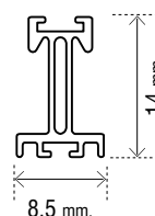
Profilo telescopico
