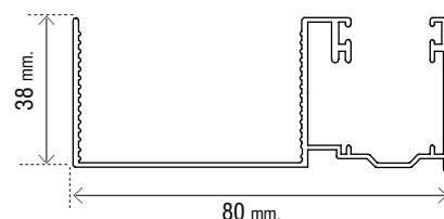
Guide con predisposizione zanzariere 80 x 38 mm.
