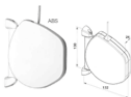
OMTACC24 Avvolgitore SHELL completo. Colore bianco.
