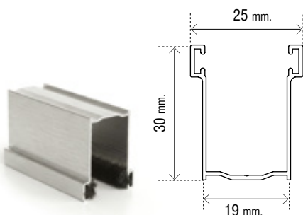
Guida in alluminio estruso 19 x 30 mm
