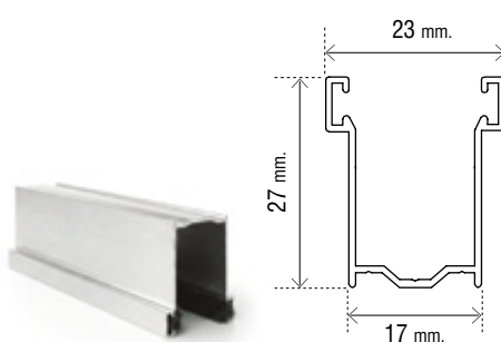
Guida in alluminio estruso 17 x 27 mm
