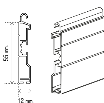
Terminali in alluminio estruso 12 x 55 mm
