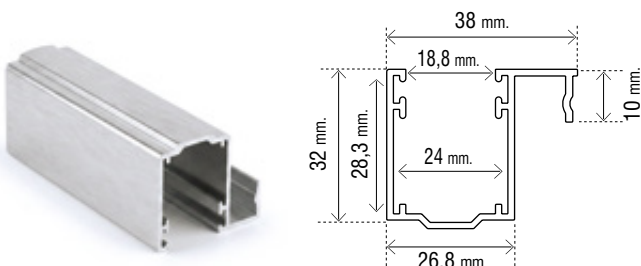
Guida in alluminio estruso 38 x 32 mm
